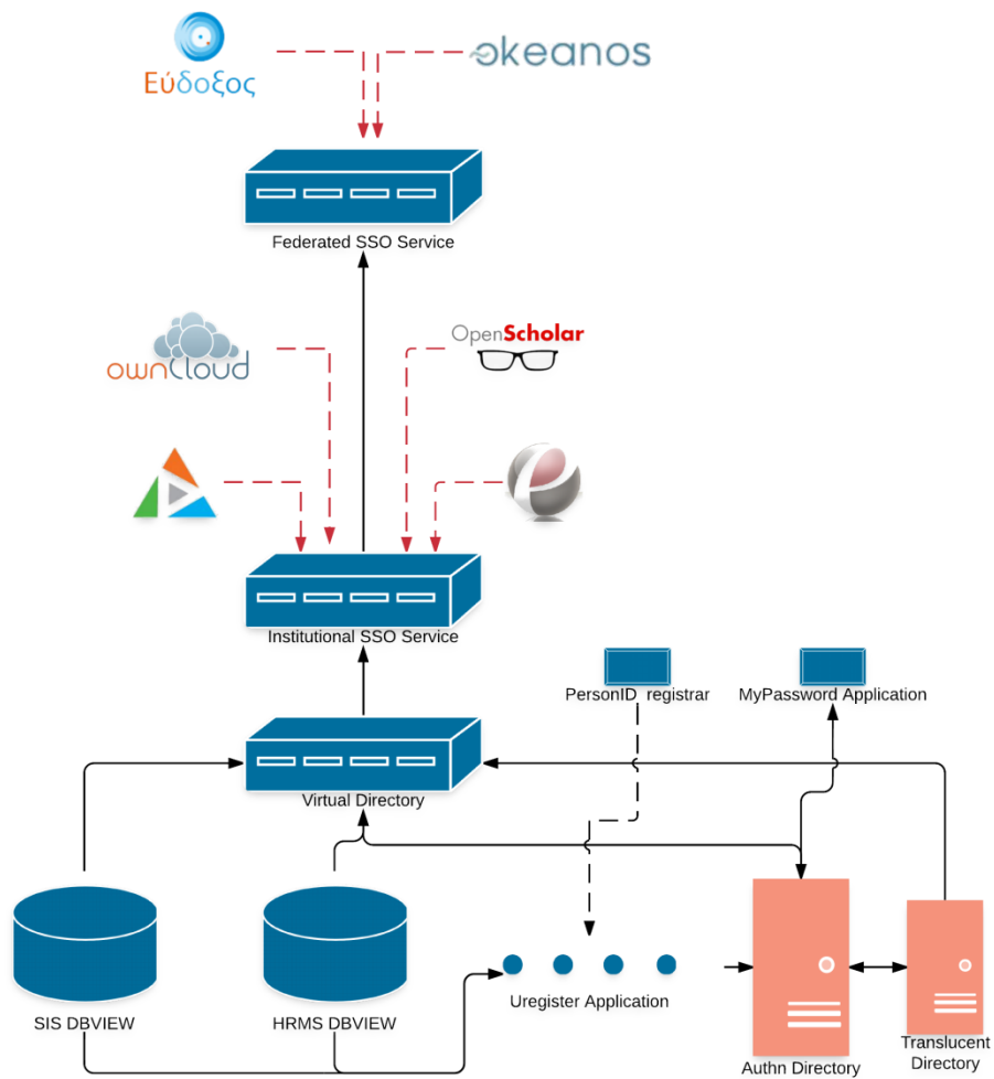
Εικόνα 2 Χωρίς IDM αλλά με διασύνδεση με trusted / authoritative users repositories
